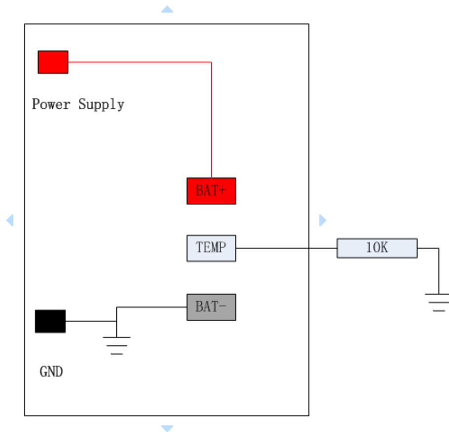
图 4.2 NTC 夹具接线方法
